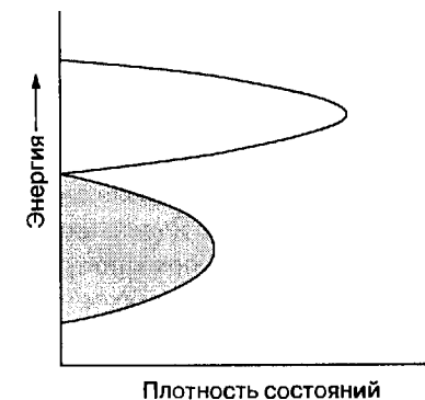
Рис. 3.52. Плотность состояний, типичная для полуметалла.
