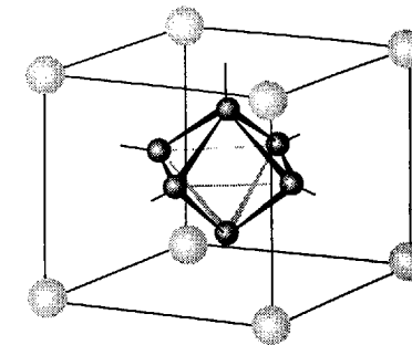
Рис. 10.8. Структура \text{CaB}_6 . Заметьте, что соседние октаэдры \text{B}_6 соединены связями между вершинами. Кристалл является аналогом \text{CsCl} , где восемь атомов Са окружают центральный октаэдр \text{B}_6 .
