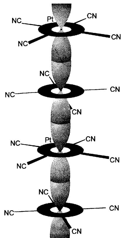
Рис. 3.54. Представление бесконечной цепочечной структуры \text{K}_2\text{Pt}(\text{CN})_4\text{Br}_{0.3} \cdot 3\text{H}_2\text{O} (КЦП) и схематическое изображение ее d -зон.
