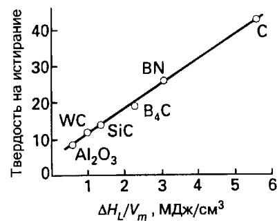
Рис. 10.6. Корреляция величины \Delta H_L/V_m и твердости вещества. Точка, относящаяся к углероду, соответствует алмазу, а точка BN — кубической фазе.
