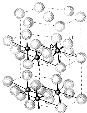
Рис. 9.24. Структура \text{CdI}_2 , которую имеют дисульфиды (в последних вместо слоев атомов иода располагаются сульфидные слои).
