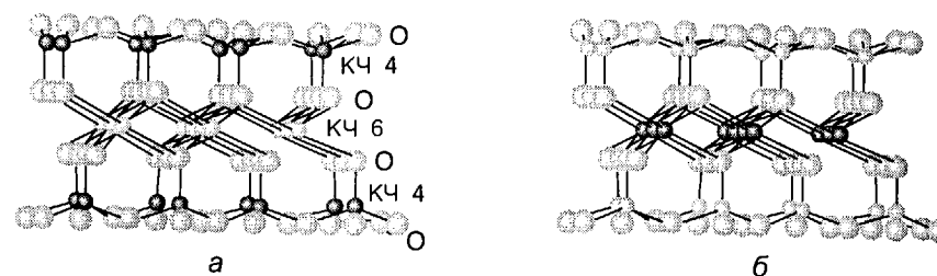
Рис. 10.28. Структура минерала мусковит (слюда, относящаяся к глинам 2 : 1) \text{KAl}_2(\text{OH})_2\text{Si}_3\text{AlO}_{10} , в которой ионы \text{K}^+ находятся между заряженными слоями (положение катионов, способных к обмену), \text{Si}^{4+} занимает позиции с координационным числом 4, а \text{Al}^{3+} — с координационным числом 6 (а); в тальке \text{Mg}^{2+} занимает места с октаэдрической координацией, а нижние атомы \text{O} замещаются группами \text{OH} (б).
