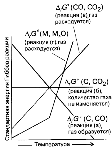
Рис. 6.2. Фрагмент диаграммы Эллингхэма, показывающий стандартные энергии Гиббса для реакции образования оксида металла и трех реакций окисления углерода. Наклон линий определяется главным образом тем, происходит ли образование или расхождение газа в ходе реакции. Фазовое превращение может приводить к появлению изломов на графиках (поскольку энтропия вещества меняется).
