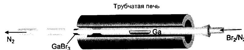
Рис. Д12.1. Трубчатая печь, используемая для синтеза безводного бромид га́ллия.
