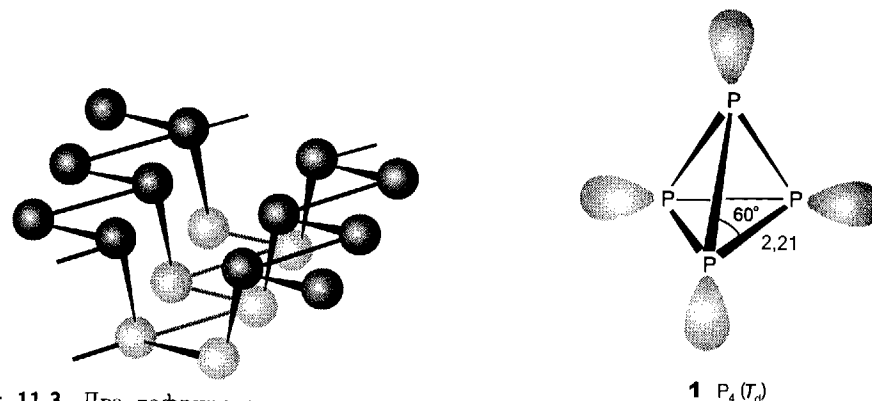
Рис. 11.3. Два гофрированных слоя черного фосфора. Следует отметить тригонально-пирамидальную координацию атомов. Темные атомы расположены ближе к наблюдателю, а более светлые — дальше.
