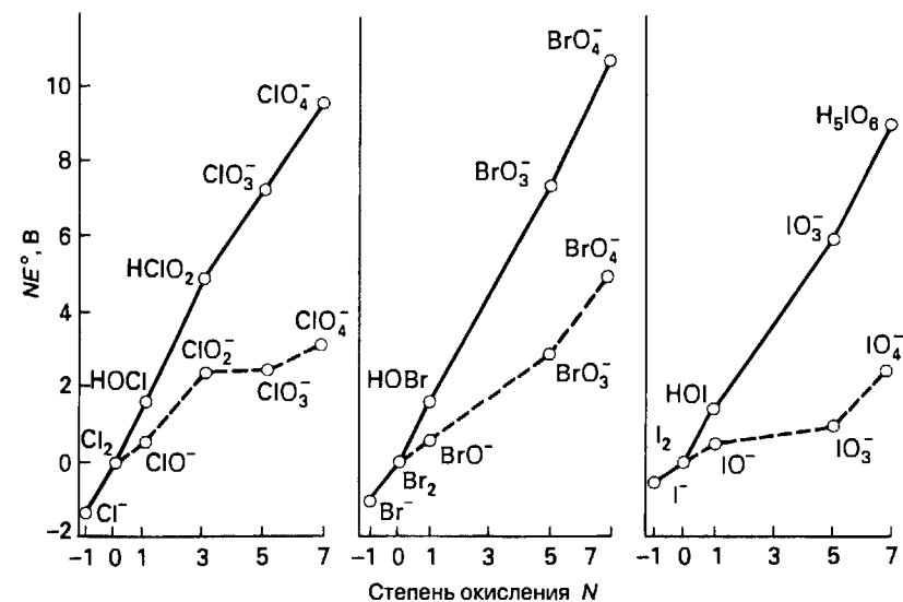
Рис. 12.14. Диаграммы Фроста для хлора, брома и йода в кислых (сплошная линия) и щелочных (пунктирная линия) растворах.
