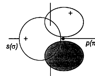
Рис. 4.19. s -Орбиталь (с \sigma -симметрией) имеет общее нулевое перекрывание с 2p_x -орбиталью (с \pi -симметрией), потому что область, где знаки орбиталей совпадают, в точности равна области, где знаки противоположны.
