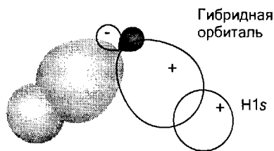
Рис. 3.37. Образование локализованных орбиталей О–Н в молекуле Н 2 О путем перекрывания гибридных орбиталей атома О с 1s-орбиталями атомов Н. Гибридные орбитали близки к sp^3 -гибридным орбиталям, показаным на рис. 3.8.
