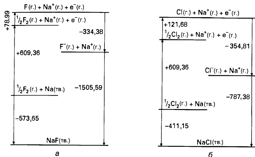
Рис. 12.1. Термохимические циклы для фторида натрия (а) и для хлорида натрия (б) (значения даны в кДж/моль).
