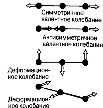
Рис. 4.25. Четыре моды нормальных колебаний молекулы \text{CO}_2 . Две деформационные моды имеют одинаковую частоту. Симметричное валентное колебание оставляет дипольный момент неизменным (равным нулю), но антисимметричное валентное и деформационные колебания приводят к изменению дипольного момента.
