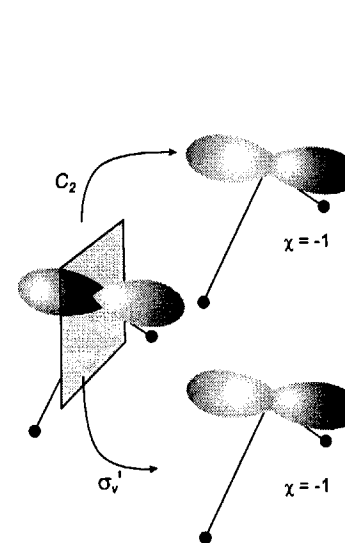
Рис. 4.16. В молекуле \text{H}_2\text{O} , относящейся к точечной группе C_{2v} , 2p_x -орбитали центрального атома меняют знак при вращении C_2 , что позволяет отнести их к типу симметрии B . Изменение знака при отражении \sigma'_v свидетельствует о том, что эта орбиталь относится к типу B_1 .
