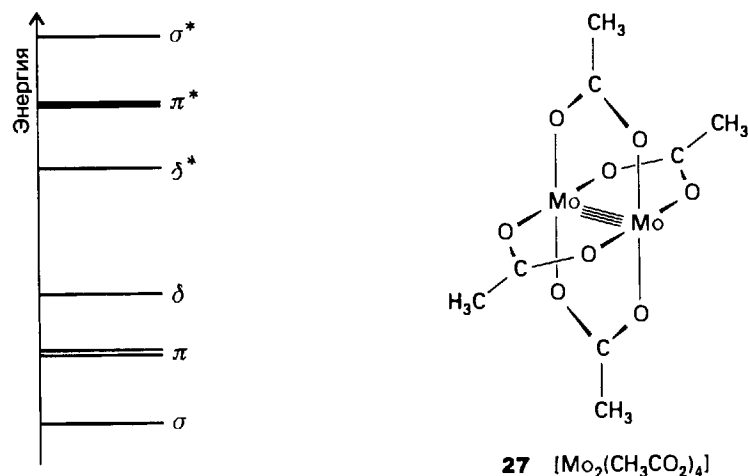
Рис. 9.21. Схематическое изображение диаграммы энергетических уровней молекулярных орбиталей для связи М–М в тетрагонально-призматическом биядерном кластере.
