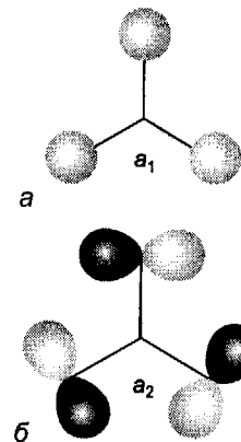
Рис. 4.14. Комбинации 1s -орбиталей атомов H, которые используются для построения молекулярных орбиталей в молекуле \text{NH}_3 . a — a_1 -Орбиталь сформирована перекрыванием показанной комбинации с 2s - и 2p_z -орбиталями атома N. б — Ни одна из валентных орбиталей азота не имеет подходящей симметрии для образования a_2 -орбитали.
