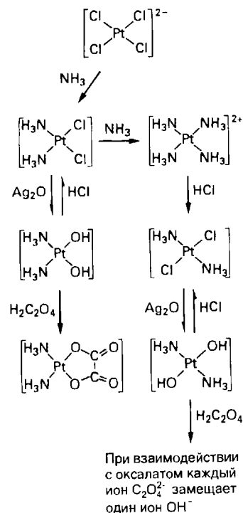
Рис. 7.1. Получение цис - и транс -дихлордиамминплатины(II) и химический метод идентификации изомеров.
