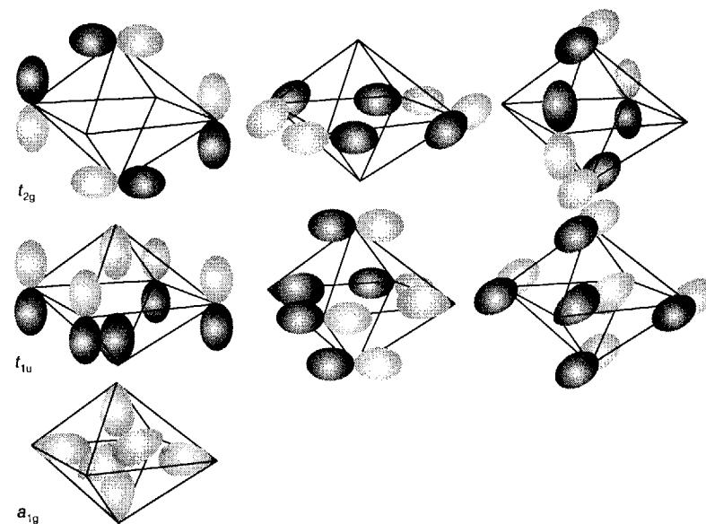
Рис. 10.9. Радиальная и тангенциальные связывающие молекулярные орбитали для [\text{B}_6\text{H}_6]^{2-} . Относительные энергии орбиталей: a_{1g} < t_{1u} < t_{2g} .
