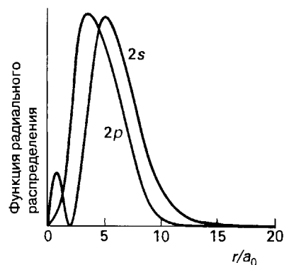
Рис. 1.12. Функции радиального распределения орбиталей водородоподобного атома. Хотя 2p-орбиталь в среднем ближе к ядру, чем 2s- (обратите внимание, где расположен ее максимум), 2s-орбиталь имеет более высокую вероятность на расстояниях, близких к ядру (с учетом внутреннего максимума).
