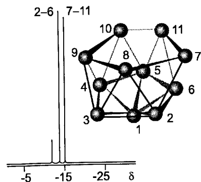
Рис. 10.13. Спектр ЯМР ^{11}\text{B} иона [\text{B}_{11}\text{H}_{14}]^- с полным подавлением спин-спинового взаимодействия с протонами. На нидо -структуру (усеченный икосаэдр) указывает соотношение интенсивностей пиков 1:5:5. [Hosmane N. S., Wermer J. R., Hong Z., Getman T. D., Shore S. G., Inorg. Chem., 26 , 3638 (1987)].
