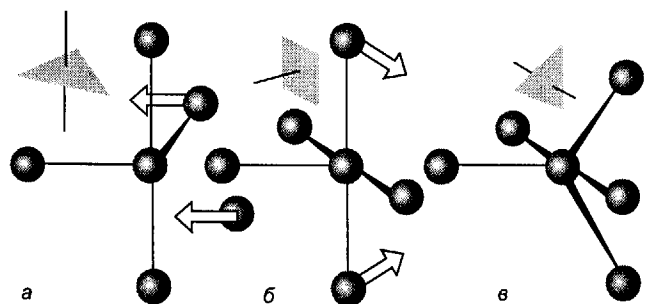
Рис. 7.3. Псевдовращение Берри, в котором тригональная бипирамида [\text{Fe}(\text{CO})_5] (а) искажается и превращается в квадратную пирамиду (б), а затем снова становится тригональной бипирамидой (в). При этом два карбонила, находящиеся первоначально в экваториальных положениях, становятся аксиальными. Примером комплекса подобного типа служит [\text{Fe}(\text{CO})_5] .
