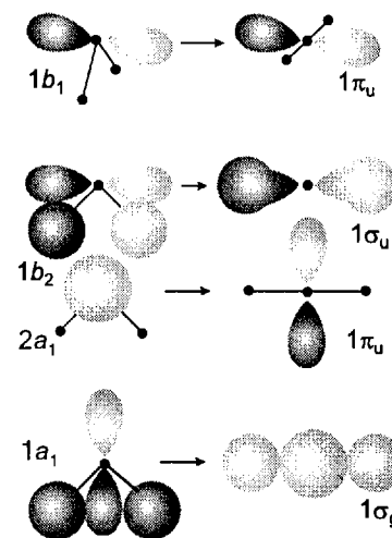
Рис. 3.40. Вид молекулярных орбиталей молекулы H_2X для двух крайних случаев корреляционной диаграммы, показанной на рис. 3.38.
