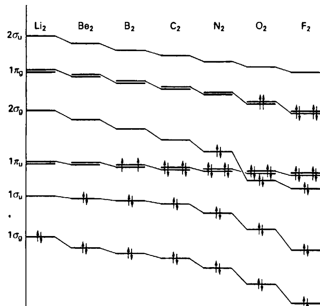
Рис. 3.17. Изменение энергии орбиталей для двухатомных гомоядерных молекул элементов второго периода до F_2 .
