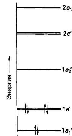
Рис. 4.30. Диаграмма энергетических уровней молекулярных орбиталей плоского иона \text{CH}_3^+ .
