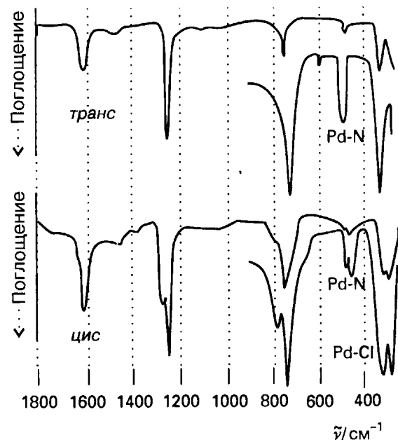
Рис. 4.27. ИК спектры цис - и транс -[Pd(NH 3 ) 2 Cl 2 ] [Layton R., Sink D. W., Durig J. R., J. Inorg. Nucl. Chem., 28, 1965 (1966)].
