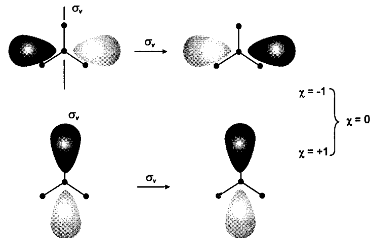
Рис. 4.20. При отражении \sigma_v 2p_x -орбиталь атома N в молекуле NH_3 меняет знак, а 2p_y -орбиталь остается неизменной. Следовательно, этой вырожденной паре соответствует характер 0 при данной операции. (Плоскость рисунка совпадает с плоскостью xy .)
