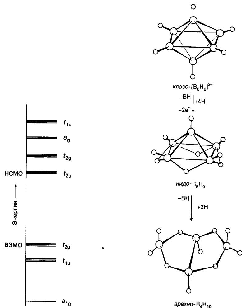
Рис. 10.11. Взаимосвязь между октаэдром \text{closo-}B_6 , квадратной пирамидой \text{nido-}B_5 и похожей на бабочку структурой \text{арачно-}B_4 .
