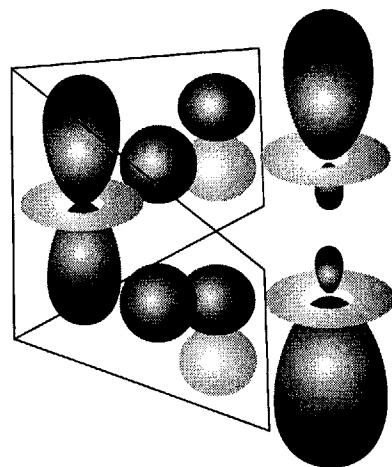
Рис. 9.23. Гибридизация s -, p_z - и d_{z^2} -орбиталей, имеющих фазы, указанные на рисунке, приводит к образованию двух расположенных вдоль одной прямой орбиталей, которые могут давать прочные \sigma -связи.
