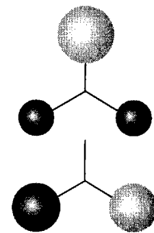
Рис. 4.15. Комбинации 1s -орбиталей атомов H, которые используются для построения e -орбиталей в молекуле \text{NH}_3 . Эти орбитали перекрываются с p_x - и p_y -орбиталями атома N.
