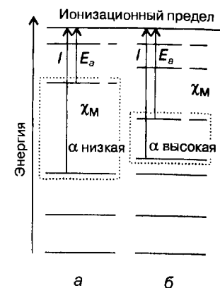
Рис. 1.26. Интерпретация электроотрицательности и поляризуемости элемента в терминах энергии граничных орбиталей (высшей заполненной и нижней свободной). Электроотрицательность высока, когда энергия этих орбиталей низкая, поляризуемость высока, когда эти орбитали расположены близко друг от друга: а — низкая \chi , низкая \alpha ; б — высокая \chi , высокая \alpha .
