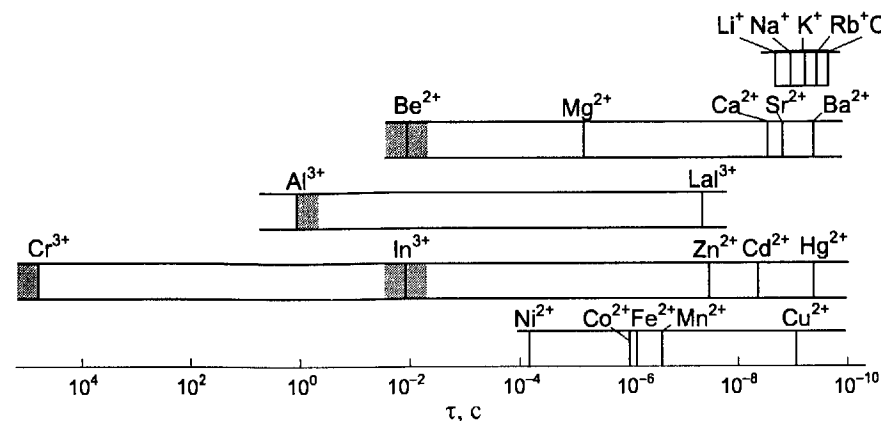
Рис. 7.25. Характеристические времена жизни комплексных акваионов металлов.
