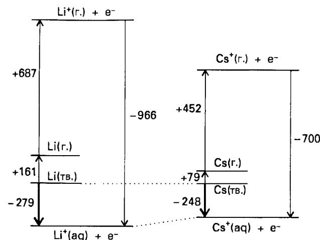
Рис. 9.6. Термодинамические циклы (энтальпия в кДж/моль) для полуреакций окисления \text{M(тв.)} \rightarrow \text{M}^+(\text{aq}) + \text{e}^- для лития и цезия. Заметим, что большая разница в энтальпии образования \text{M}^+(\text{г.}) компенсируется соответствующим изменением энтальпии гидратации \text{M}^+ .
