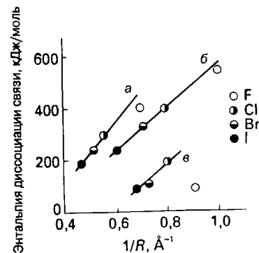
Рис. 12.6. Зависимость энтальпии диссоциации связи от обратной длины связи: а — углерод-галоген, б — водород-галоген, в — галоген-галоген. Следует отметить слабость связи \text{X}-\text{F} . [Politzer P., J. Am. Chem. Soc., 91, 6235 (1969)].
