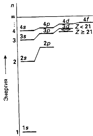
Рис. 1.19. Диаграмма энергетических уровней многоэлектронного атома с Z < 21 (до кальция). Для элементов, расположенных за скандием, наблюдается изменение в порядке расположения уровней. Эта диаграмма поясняет основной принцип заполнения электронных оболочек (разд. 1.7) с учетом того, что только два электрона могут занимать каждую орбиталь.
