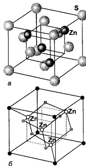
Рис. 2.12. Структура сфалерита (цинковой обманки) (два способа изображения). Заметим ее сходство с ГЦК структурой на рис. 2.5, в которой половина тетраэдрических пустот занята катионами \text{Zn}^{2+} .
