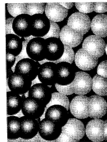
Рис. 12.7. Твердые хлор, бром и йод имеют одинаковое строение, однако взаимодействие между ближайшими не связанными в молекулу атомами слабее для \text{Cl}_2 и \text{Br}_2 по сравнению с \text{I}_2 [Donohue J., The structures of the elements. Wiley, New York, 1974].
