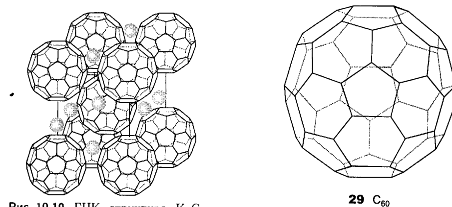
Рис. 10.19. ГЦК структура K_3C_{60} . Показан только фрагмент элементарной ячейки.
