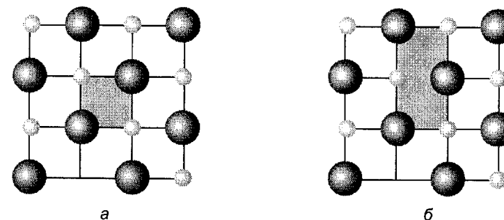
Рис. 2.1. Двумерная структура и два варианта выбора элементарной ячейки. Весь кристалл можно получить параллельным переносом любой из этих ячеек, но вариант (а) предпочтительнее, так как он обладает максимальной симметрией, в то время как вариант (б) — нет.
