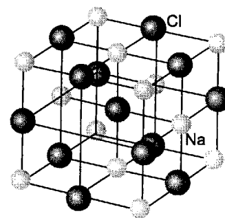
Рис. 2.10. Структура каменной соли. Обратите внимание на сходство с ГЦК структурой на рис. 2.4 с анионами в каждой октаэдрической пустоте. С другой стороны, можно рассматривать ГЦК упаковку анионов с катионами в каждой октаэдрической пустоте.
