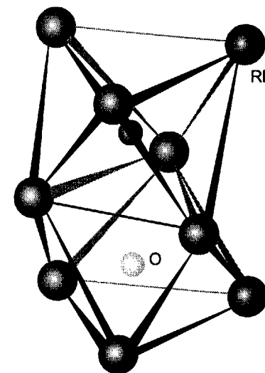
Рис. 9.8. Структура \text{Rb}_9\text{O}_2 . В этом кластере каждый атом O находится в центре октаэдра из атомов Rb.
