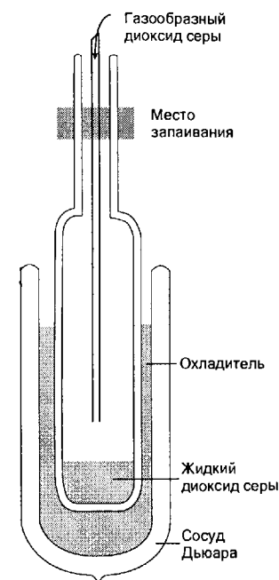
Рис. Д11.2. Конденсация диоксида серы в трубке Кариуса.
