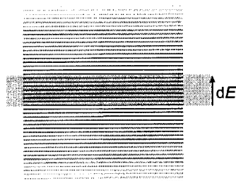
Рис. 3.50. Плотность состояний — отношение количества энергетических уровней в бесконечно малой области зоны к ширине этого участка ( dE ).
