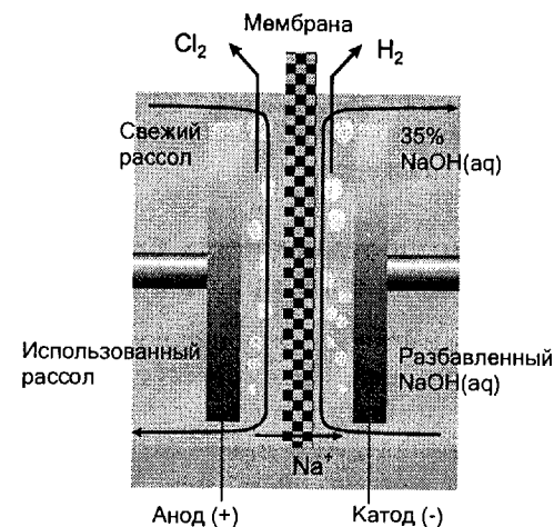
Рис. 12.3. Схематическое изображение современного электролизера для производства хлора с использованием катионообменной мембраны, которая высокопроницаема для иона \text{Na}^+ и почти непроницаема для ионов \text{Cl}^- и \text{OH}^- .
