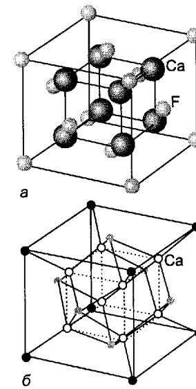
Рис. 2.13. Структура флюорита (два способа изображения). Структура имеет ГЦК упаковку катионов, в которой анионы занимают все тетраэдрические пустоты. С другой стороны, эту структуру можно рассматривать как примитивную кубическую решетку анионов, в которой половина кубических пустот занята катионами.
