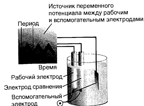
Рис. Д6.1. Схема эксперимента циклической вольтамперометрии. Каждый период изменяемого со временем потенциала (первый период обозначен вертикальными линиями) отвечает одному полному циклу циклической вольтамперограммы (на двух следующих рисунках).
