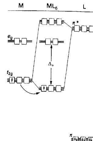
Рис. 7.23. Лиганды, действующие как \pi -акцепторы, увеличивают \Delta_o .
