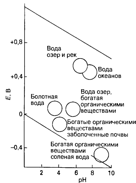
Рис. 6.14. Область устойчивости воды, на которой показаны интервалы значений pH — потенциал, характерные для различных природных вод.
