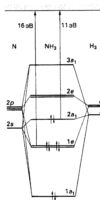
Рис. 3.33. Диаграмма энергетических уровней молекулярных орбиталей молекулы \text{NH}_3 с экспериментально найденными значениями углов \text{HNN} ( 107^\circ ) и длин связей.
