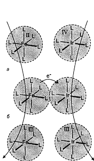
Рис. 6.6. Схематическое представление внешней сферной окислительно-восстановительной реакции: а — реагирующие ионы диффундируют друг к другу через растворитель, и в тот момент, когда они находятся в контакте, происходит перенос электрона от одного иона к другому; б — продукты затем диффундируют друг от друга. В результате реакции координационное окружение ионов остается неизменным (изображено в виде заштрихованных сфер). Поскольку меняется радиус центрального иона металла, то могут происходить небольшие изменения длин связей металл–лиганд.
