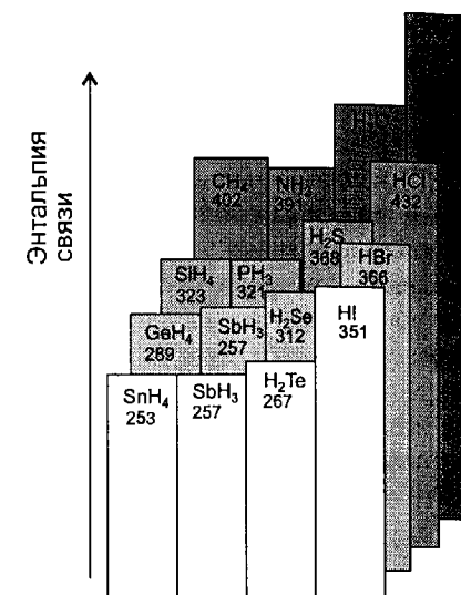
Рис. 8.11. Средние энтальпии связи (кДж/моль) при 298 К.
