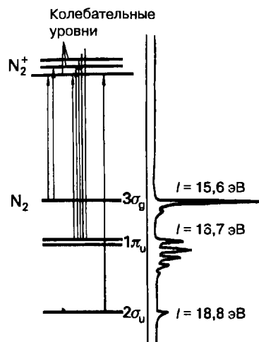
Рис. 3.13. УФ фотоэлектронный спектр молекулы N_2 . Тонкая структура спектра возникает вследствие возбуждения колебаний в катине, образующемся в результате выбивания электрона.
