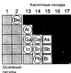
Рис. 5.4. Элементы, символы которых обведены в кружок, даже в высших степенях окисления образуют амфотерные оксиды. Элементы, символы которых помещены в квадраты, в высших степенях окисления образуют кислотные оксиды, а в низших — амфотерные.
