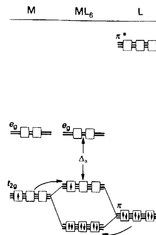
Рис. 7.22. Влияние \pi -связывания на параметр расщепления \Delta_o лигандов. Лиганды, действующие как \pi -доноры, уменьшают \Delta_o .
