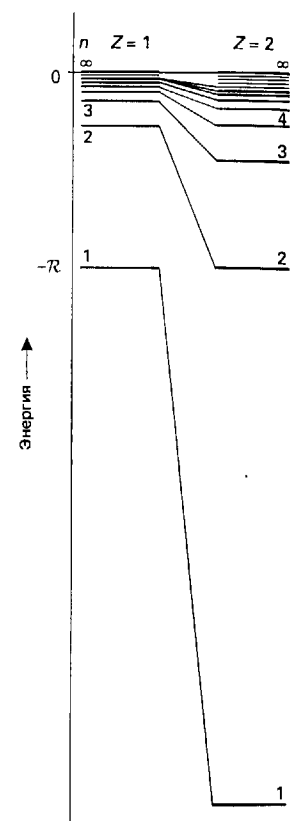
Рис. 1.7. Квантованные энергетические уровни атома водорода H ( Z = 1 ) и иона гелия He^+ ( Z = 2 ). Энергия водородоподобного атома пропорциональна Z^2 .
