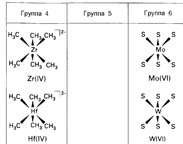
Обобщающая схема 4. Тригонально-призматические комплексы
