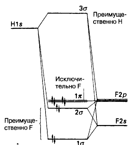
Рис. 3.21. Диаграмма энергетических уровней молекулярных орбиталей молекулы HF. Относительное положение атомных орбиталей отражает энергии ионизации атомов.
