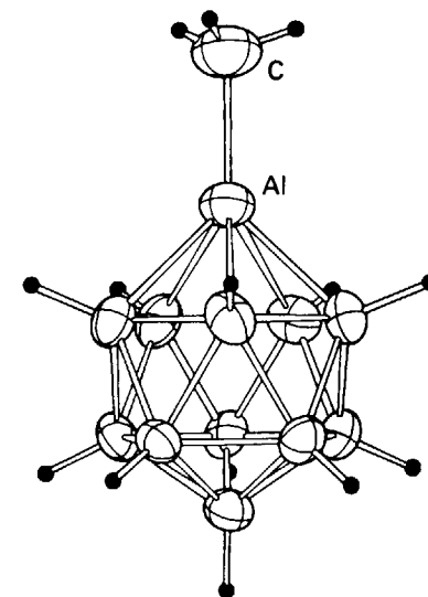
Рис. 10.14. Структура икозо - [\text{B}_{11}\text{H}_{11}\text{AlCH}_3]^{2-} [Getman T. D., Shore S. G., Inorg. Chem., 27 , 3439–40 (1998)].
