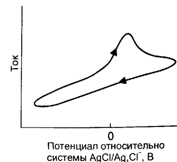
Рис. Д6.3. Циклическая вольтамперограмма для реакции, которая в одном направлении простая, а в обратном — сложная. Волна восстановления отсутствует.
