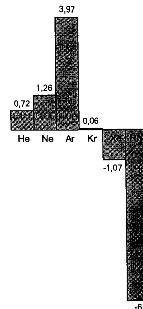
Рис. 12.15. Распространенность благородных газов в земной коре (приведены десятичные логарифмы распространенности в миллионных долях по объему в атмосфере) [Emsley J., The elements. Oxford University Press (1998)].
