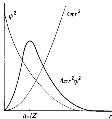
Рис. 1.11. Функция радиального распределения 1s-орбитали водородоподобного атома. Произведение выражения 4\pi r^2 (которое увеличивается с увеличением r ) и \psi^2 (которая экспоненциально уменьшается) проходит через максимум при r = a_0/Z .
