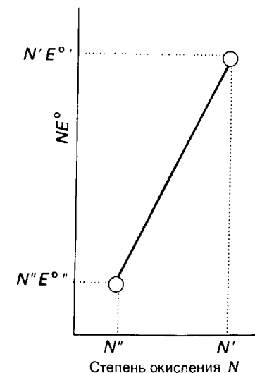
Рис. 6.11. Общий вид части диаграммы Фроста, используемой для установления взаимосвязи между наклоном прямой и стандартным потенциалом соответствующей пары.
