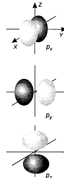
Рис. 1.14. Граничные поверхности p-орбиталей. Каждая из них имеет одну узловую плоскость, проходящую через ядро. Например, для p_z узловой плоскостью будет плоскость xy . Светлые участки соответствуют областям с положительной амплитудой, а темные — с отрицательной.
