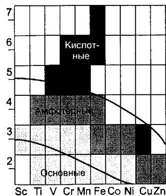
Рис. 5.5. Влияние степени окисления на кислотно-основной характер оксидов элементов первого ряда переходных металлов. Степени окисления, для которых характерны кислотные оксиды, показаны темным цветом, а для которых характерны основные оксиды — светло-серым цветом. При степенях окисления, расположенных между двумя кривыми, оксиды являются амфотерными.
