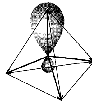
Рис. 3.8. Четыре эквивалентные sp^3 -гибридные орбитали. Каждая направлена к вершине правильного тетраэдра.
