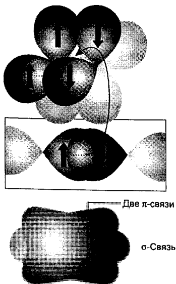
Рис. 3.6. Описание молекулы азота по методу ВС: два электрона образуют \sigma -связь, а оставшиеся две пары образуют \pi -связи. В линейных молекулах, где не определено направление осей x и y , электронная плотность \pi -связей имеет цилиндрическую симметрию относительно оси, проходящей через ядра атомов.
