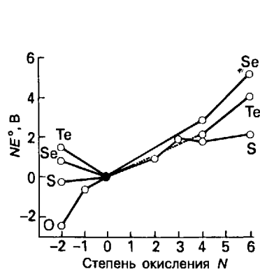
Рис. 11.6. Диаграмма Фроста для элементов группы кислорода в кислой среде. Степени окисления -2 соответствуют соединениям H_2E , степени окисления -1 — H_2O_2 . Положительные степени окисления относятся к оксидам или оксокислотам: для S(II) — это тиосульфат S_2O_3^{2-} , а для S(III) — гидродитионит HO_2SSO_2^- .
