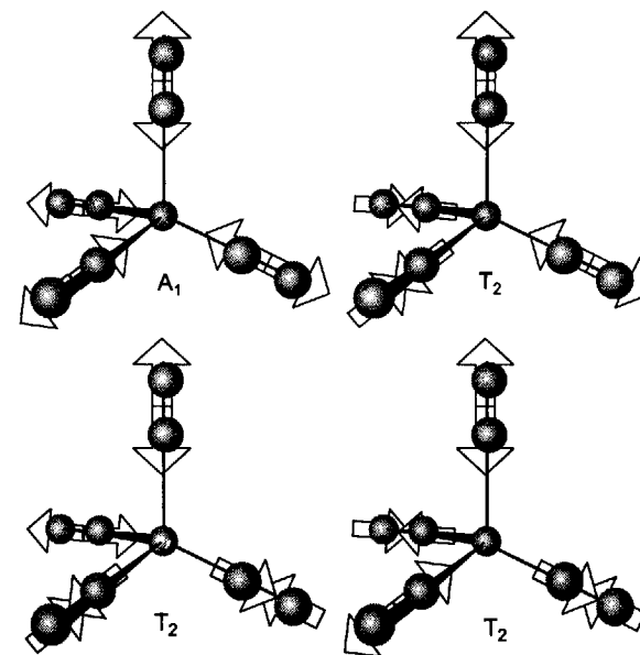
Рис. 4.28. Моды молекулы Ni(CO) 4 , которые соответствуют валентным колебаниям в группах CO. Мода A_1 невырождена, моды T_2 трехкратно вырождены. (Сравните относительные фазы смещений с относительными фазами СЛК аналогичной симметрии в приложении 4.)
