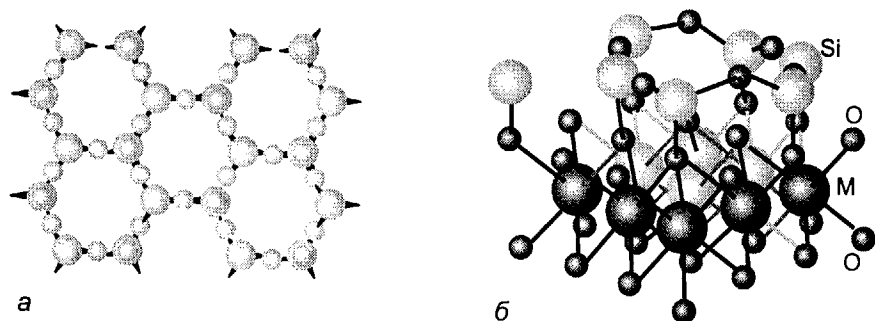
Рис. 10.27. Сетка тетраэдров \text{SiO}_4 с атомами \text{O} над каждым атомом \text{Si} , вид сверху (а); вид сбоку на сетку, где слои \text{Si/O} соединены с сеткой октаэдров \text{MO}_6 (б). Это структура минерала хризотила, где \text{M} = \text{Mg} . Когда \text{M} означает \text{Al}^{3+} и каждый атом внизу замещен группой \text{OH} , эта структура соответствует минералу каолиниту, глине 1 : 1.
