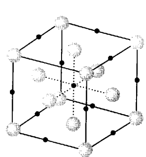
Рис. 2.4. Расположение октаэдрических пустот относительно атомов в ГЦК структуре. Пустоты называют по относительным позициям узлов решетки, расположенным вокруг них.
