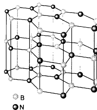
Рис. 10.4. Слоистая гексагональная структура нитрида бора. Следует отметить, что кольца расположены друг под другом.
