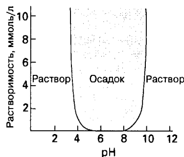
Рис. 5.7. Зависимость растворимости \text{Al}_2\text{O}_3 от pH (выражена через общую концентрацию \text{Al} ). В сильнокислом растворе алюминий присутствует в виде [\text{Al}(\text{OH}_2)_6]^{3+} , а в сильнощелочном — в виде [\text{Al}(\text{OH})_4]^- .
