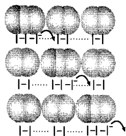
Рис. 12.13. Одна из возможных моделей переноса заряда вдоль полииодидной цепи, где эффективное перемещение иона I^- объясняется обменом коротких и длинных связей. Показаны три последовательные стадии перемещения. Как и при переносе протона во льду или в воде, иодид-ион из иона I_3^- слева не тот, что появляется справа.
